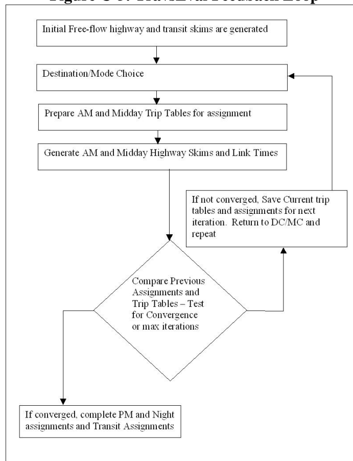
Figure C-5: TravsEval Feedback Loop
